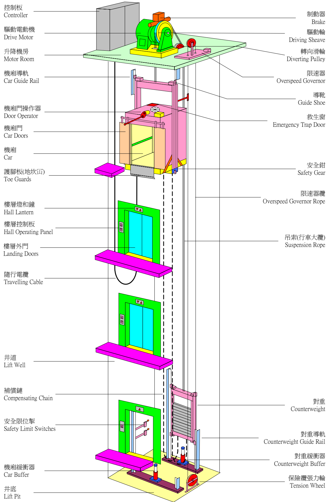
升降機的設備與構造立體圖
