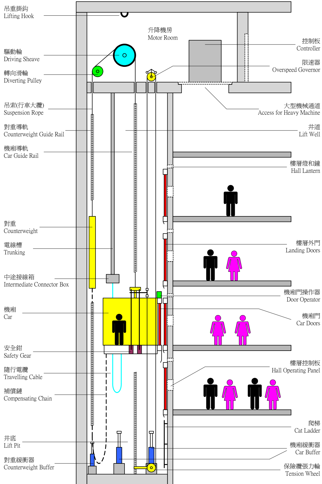
升降機的設備與構造平面圖
